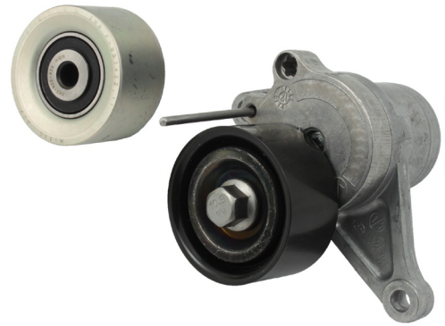
Kuva 1: Metallinen kiristin- ja ohjainrulla
